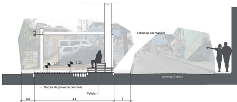
Fig.36: CORTE AA'. Desenho do As-Built. Imagem feita pelos alunos/2015.
