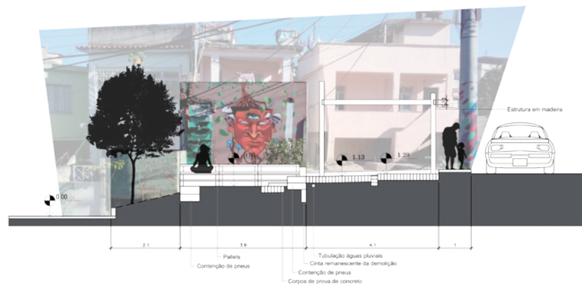
Fig.37: CORTE BB'. Desenho do As-Built. Imagem feita pelos alunos/2015.
